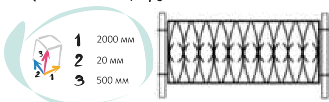
16008 Газонное ограждение со столбом ГОЛ8 (500x2000 мм), грунтовка
