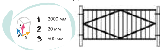
16003 Газонное ограждение со столбом ГОЛ3 (500x2000 мм), грунтовка
