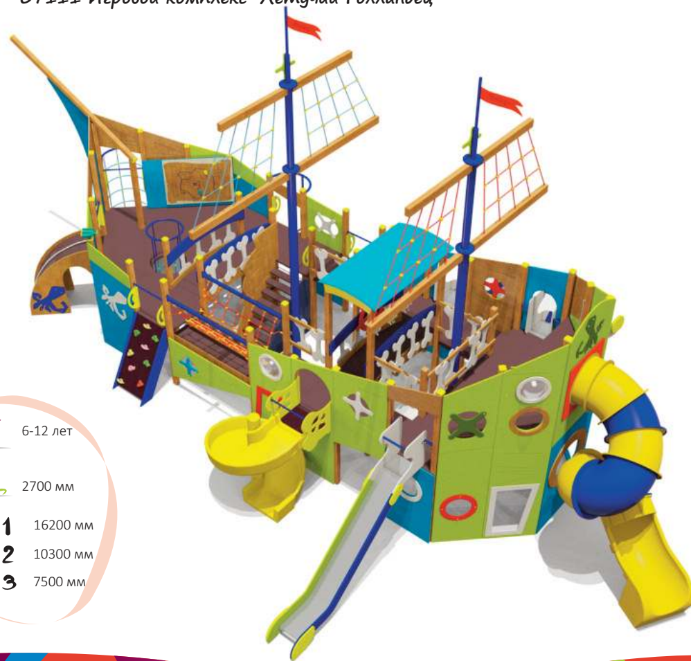
07111 Игровой комплекс "Летучий Голландец"
