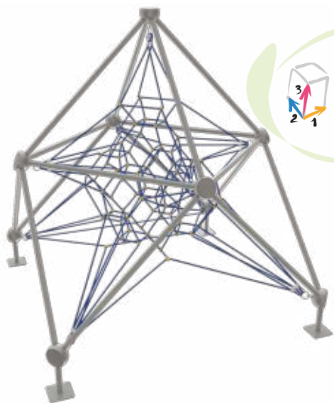
Канатная конструкция СОКРАТ КН-00228
