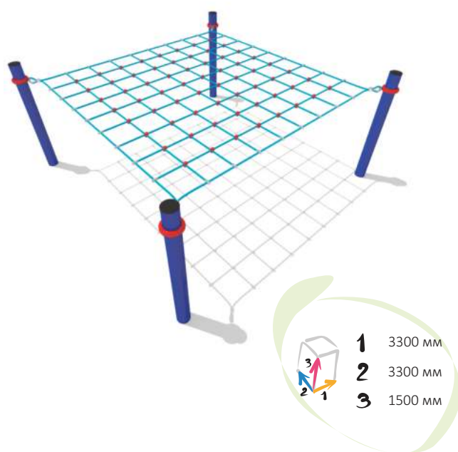
33104 Канатная конструкция
