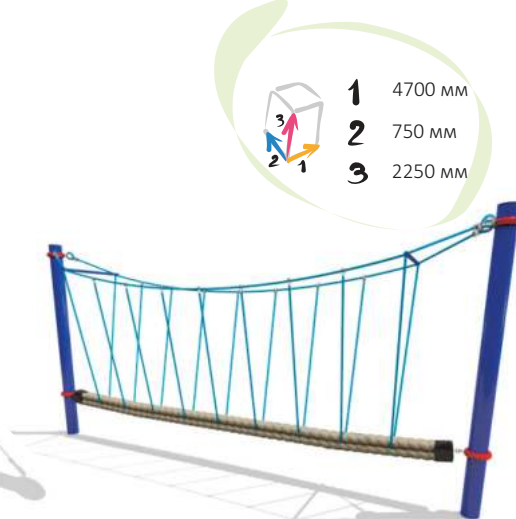
33210 Канатная конструкция
