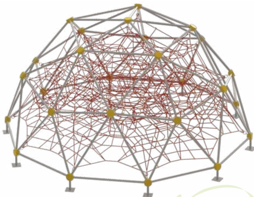
Канатная конструкция СОКРАТ КН-00851
