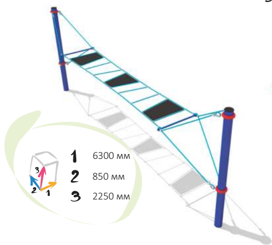
33202 Канатная конструкция
