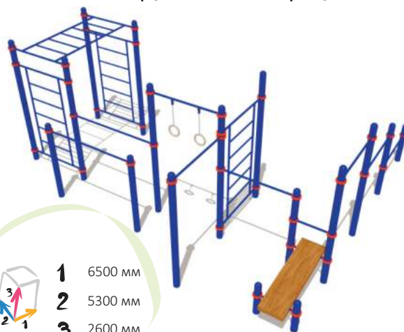
25022 Оборудование для Воркаут
