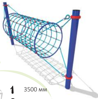
33002 Канатная конструкция
