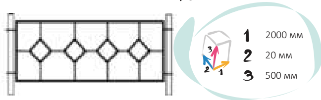
16010 Газонное ограждение со столбом ГОЛ10 (500x2000 мм), грунтовка
