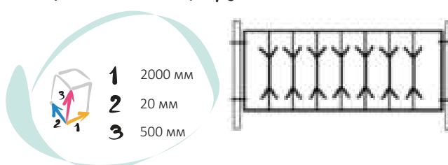
16007 Газонное ограждение со столбом ГОЛ7 (500x2000 мм), грунтовка
