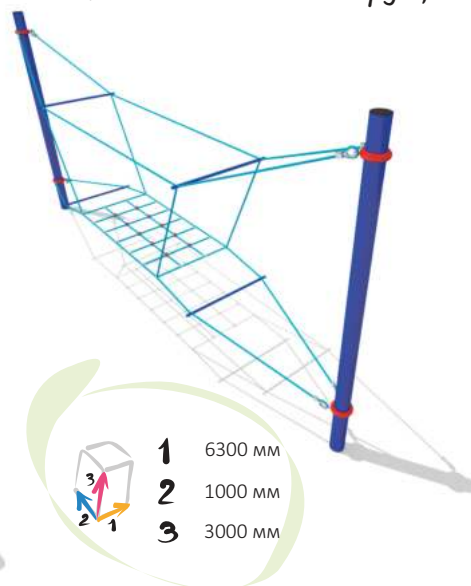
33204 Канатная конструкция
