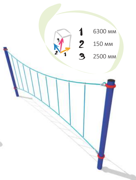
33206 Канатная конструкция
